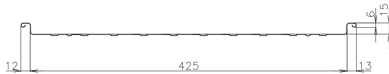
A - A 断面図
