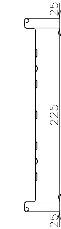
B - B 断面図
