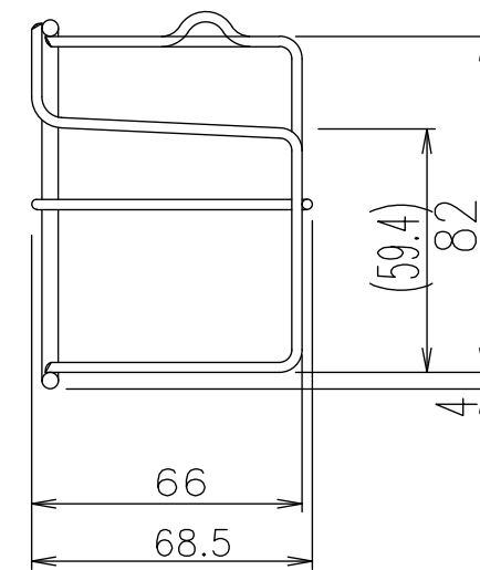
A - A 断面図
